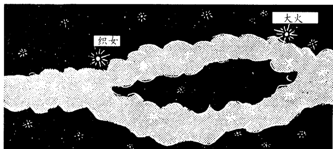
图 112 向银心看去，给人的感觉是这条神话中的河分成两叉
