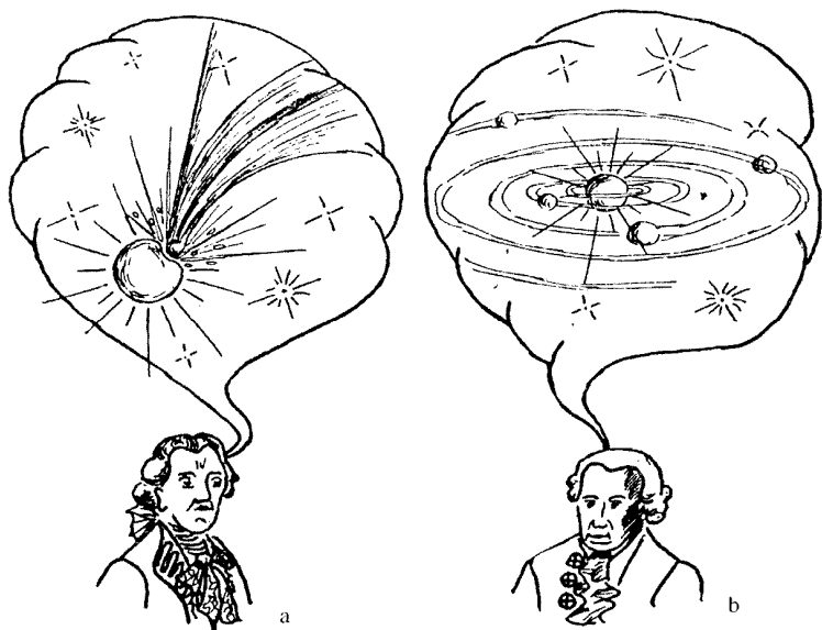
图 117 宇宙论的两种学派 a. 布丰的碰撞说；b. 康德的气体环说
