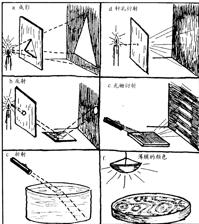
图 55 左边三个图是可以光线来解释的现象， 右边三个图是无法用光线解释的现象
