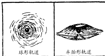
图 54 原子内电子运动的微观光学图景
