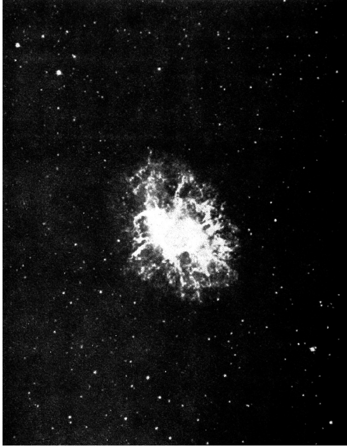
图版Ⅷ 蟹状星云。中国古代天文学家在 1054 年在这个星云的位置上观测到一颗超新星爆炸，这个星云是爆发时抛出的气体膨胀而成的包层
