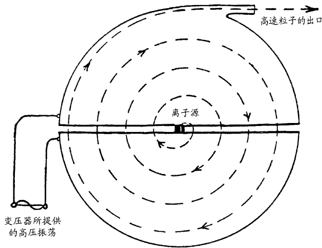
图 70 回旋加速器的原理
