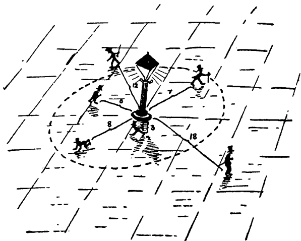
图 81 灯柱附近六名醉鬼的统计分布情况
