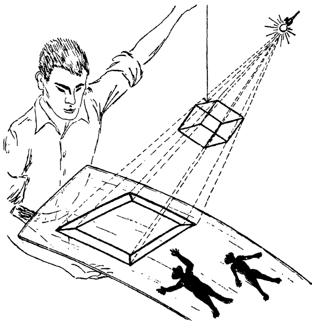
图 25 二维扁片人正惊奇地观察着三维立方体在他们那个世界上的投影
