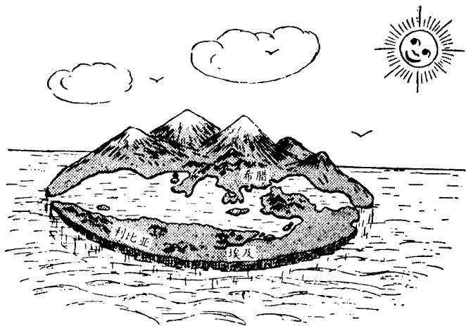
图 104 古代人认为世界只有这么大
